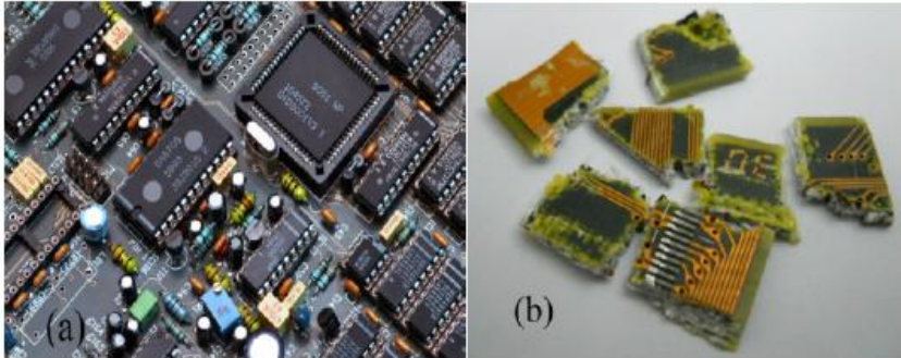
(a) PCB einer Computer-Hauptplatine (b) nach dem Schneiden
