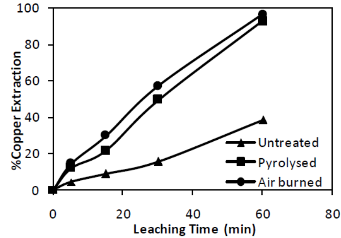
Auswirkung der thermischen Vorbehandlung auf die Metallgewinnung mit der Zeit
